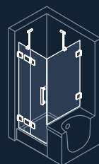
Kridlové dvere SOLVA zalamovacie do niky šírka 500~1250 mm, výška 1200~2000 mm, hlbka no limit
